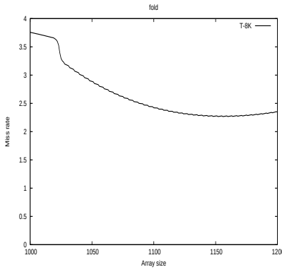
(d) fold 8K Traditional
