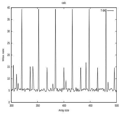
(d) calc 8K Traditional
