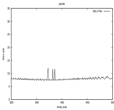
(h) jacobi 2 \times 4K Color
