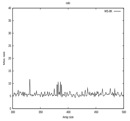
(f) calc 1x8K Color
